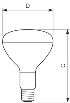
R125 IR 375W E27 230-250V CL
